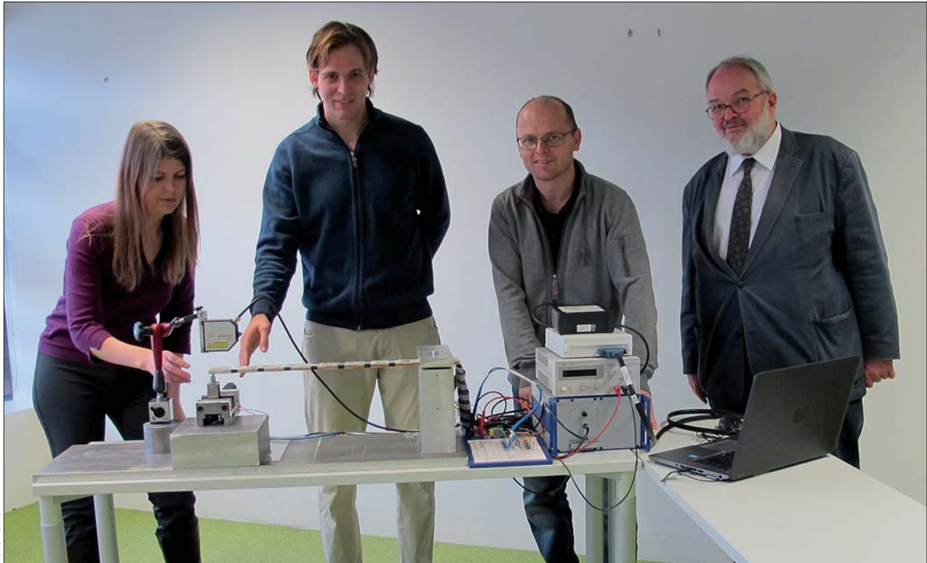
Die Versuchsanordnung – ein Metallbalken wird zu Schwingungen angeregt: auf dem Balken sind piezoelektrische Elemente angebracht, die über elektrische Schaltkreise miteinander verbunden sind (v.l.: Buchberger, Schöftner, Brandl, Irschik)
