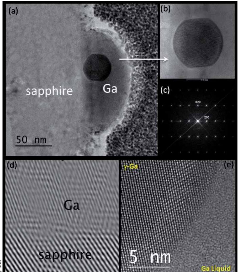
Aufnahmen unter dem Transmissionselektronenmikroskop. Gallium in Saphir (a); Großaufnahme von Gallium (b) und Reflektionen eines Galliumkristalls (c)
