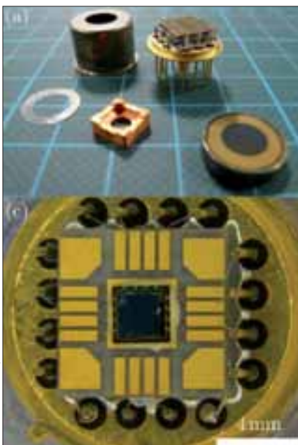
Das »Innenleben« der neuartigen Wärmebildkamera
