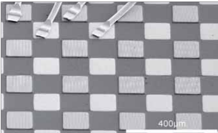
Pixel-Array für die Aufnahme von Wärmebildern, entwickelt an der TU Wien.
