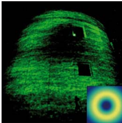
Eine Lichtschraube an der Wand des Optical Ground Station Teleskops der ESA in Teneriffa, Kanarische Inseln – nach mehr als 100 Kilometern Transmission. Man erkennt klar eine ringförmige Struktur, ein Merkmal dieser Lichteigenschaft.
