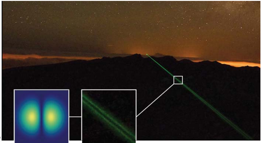
Eine Lichtschraube am 143 Kilometer langen Weg zwischen den Kanarischen Inseln von La Palma nach Teneriffa
