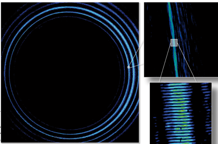
Kameraaufnahme in Falschfarbendarstellung eines Lasers, der sich in einer quantenmechanischen Überlagerung aus den Quantenzahlen +10000 und -10000 befindet. Erst der doppelte Zoom zeigt die enorme Komplexität der Lichtstruktur.
