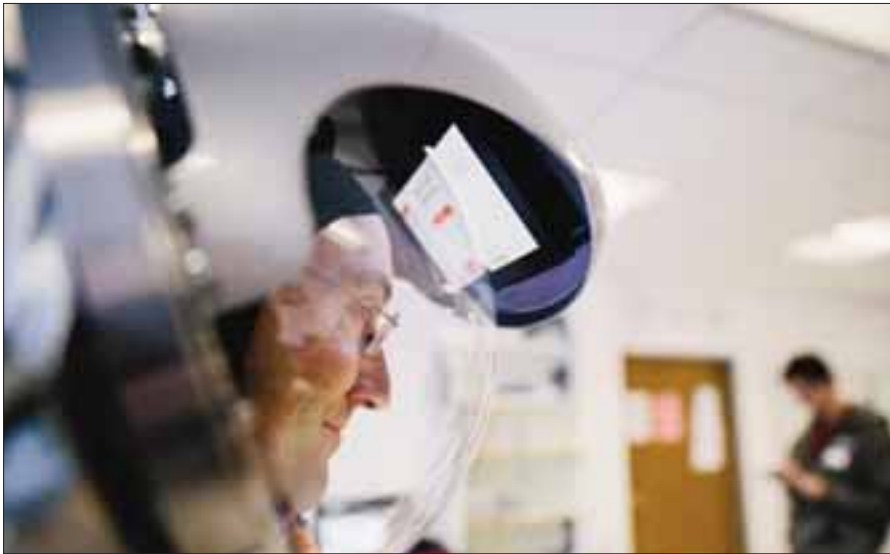
Die Sensoren des Lebenserhaltungssystems des Raumanzuges werden im Labortest vermessen, hier die Temperaturfühler im Anzug.
