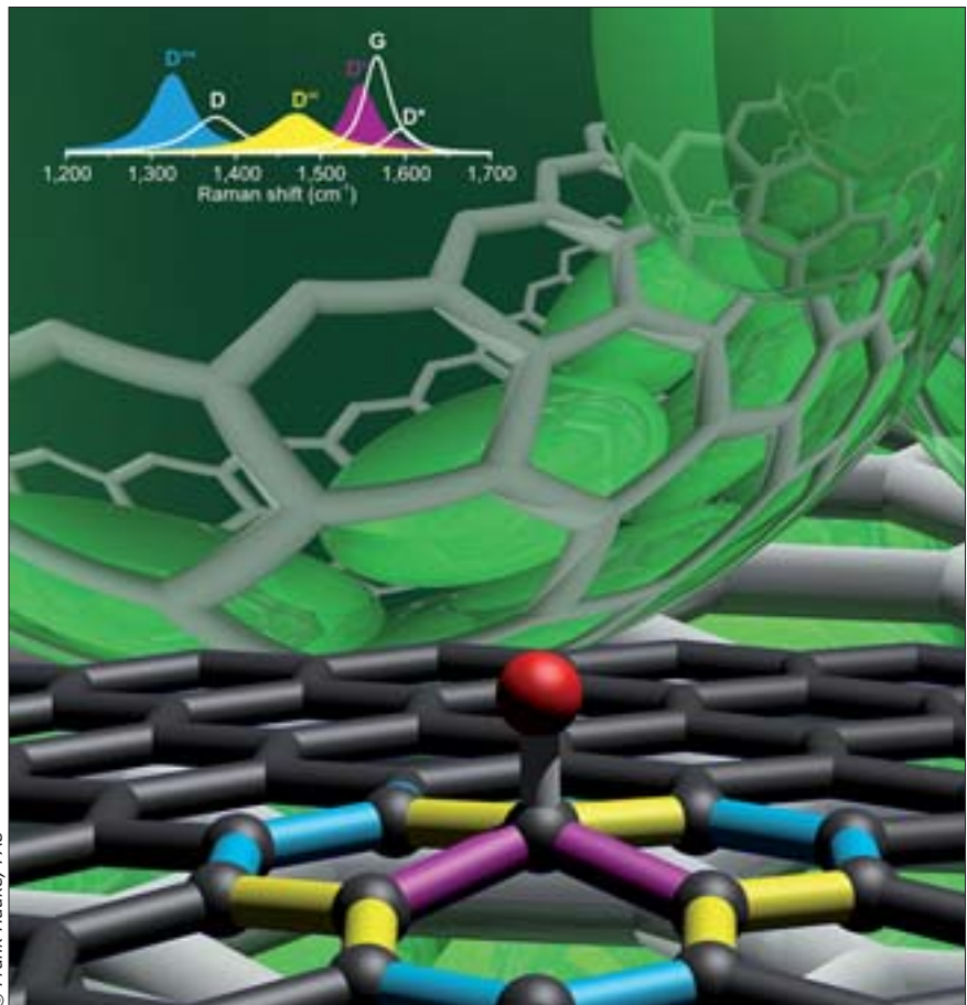
Ausschnitt aus dem Graphen-Netzwerk mit chemisch gebundenem Wasserstoffatom: Die spektrale Schwingungssignatur der einzelnen Kohlenstoff-Kohlenstoff Bindungen in direkter Nachbarschaft zum gebundenen Wasserstoffatom sind farbig gekennzeichnet
