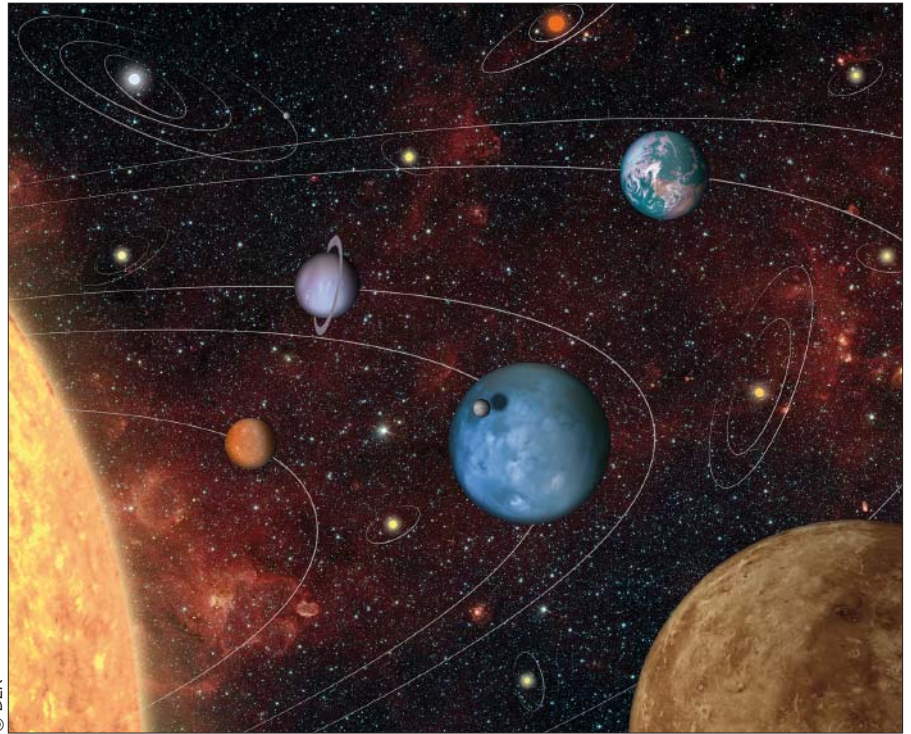
Künstlerische Interpretation eines fremden Planetensystems
