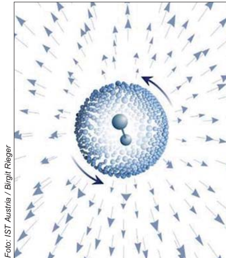
Das suprafluide Heliumtröpfchen wirkt wie ein magnetischer Monopol.
