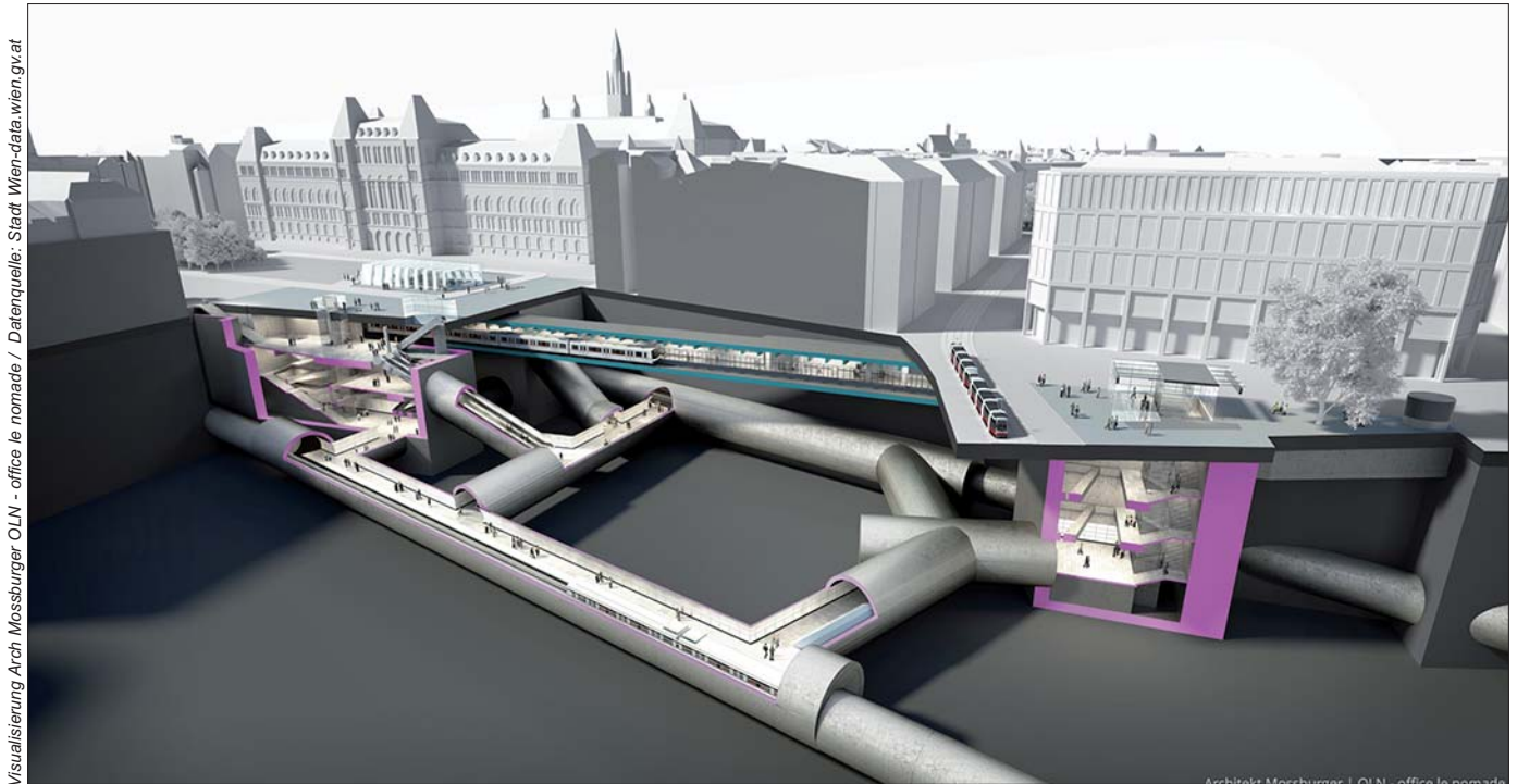
3D-Visualisierung der zukünftigen Knotenstation Rathaus von U2 und U5
