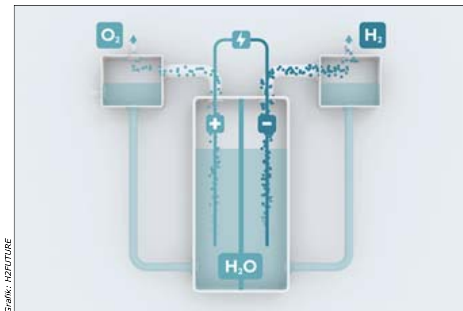
Der H2FUTURE-Prozess: Wasserstoff, gewonnen aus CO 2 -freiem Grünstrom, stellt ein gewaltiges Potential für den Einsatz als Industrirohstoff wie auch zur Energiespeicherung dar.
