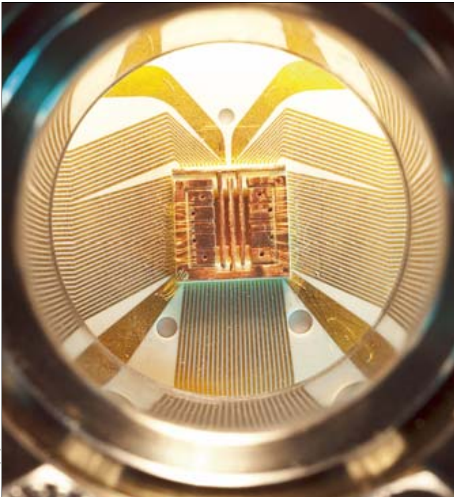
Miniaturisierte Ionenfalle am IQOQI Innsbruck für den gleichzeitigen Einsatz verschiedener Ionenstränge zur Quanteninformationsverarbeitung.
