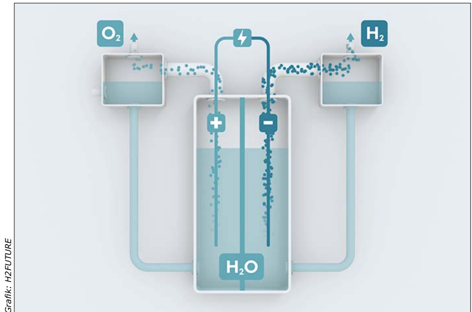
Der H2FUTURE-Prozess: Wasserstoff, gewonnen aus CO 2 -freiem Grünstrom, stellt ein gewaltiges Potential für den Einsatz als Industrierohstoff wie auch zur Energiespeicherung dar.
