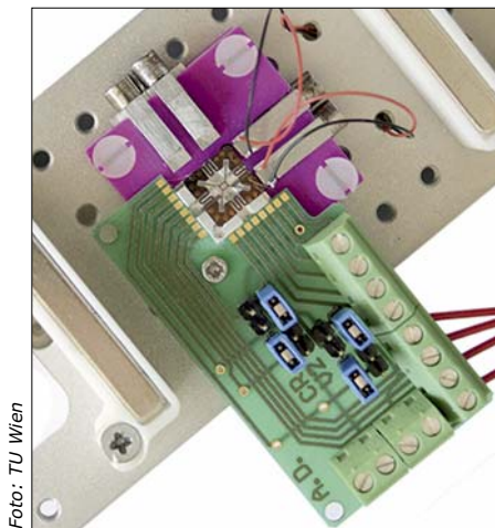
Der neuartige Kraft-Sensor der TU Wien
