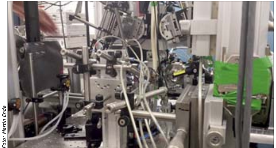
Experimentalaufbau des verwendeten Laserheizsystems für Diamantstempelzellen an der Strahllinie ID27 am ESRF
