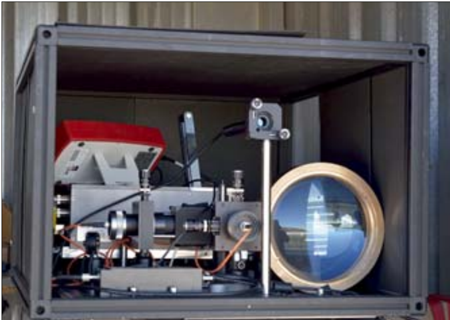
Eine der zwei mobilen Empfangsstationen für verschränkte Photonen, die von den Quantenphysikern der Österreichischen Akademie der Wissenschaften (ÖAW) auf La Palma für die Messung der Verschränkung eingesetzt wurde.
