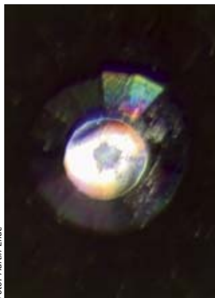
Mikroskopaufnahme durch einen der beiden Stempeldiamanten auf das auf 27 GPa komprimierte feste CO 2 (dunkler Fleck Bildmitte)
