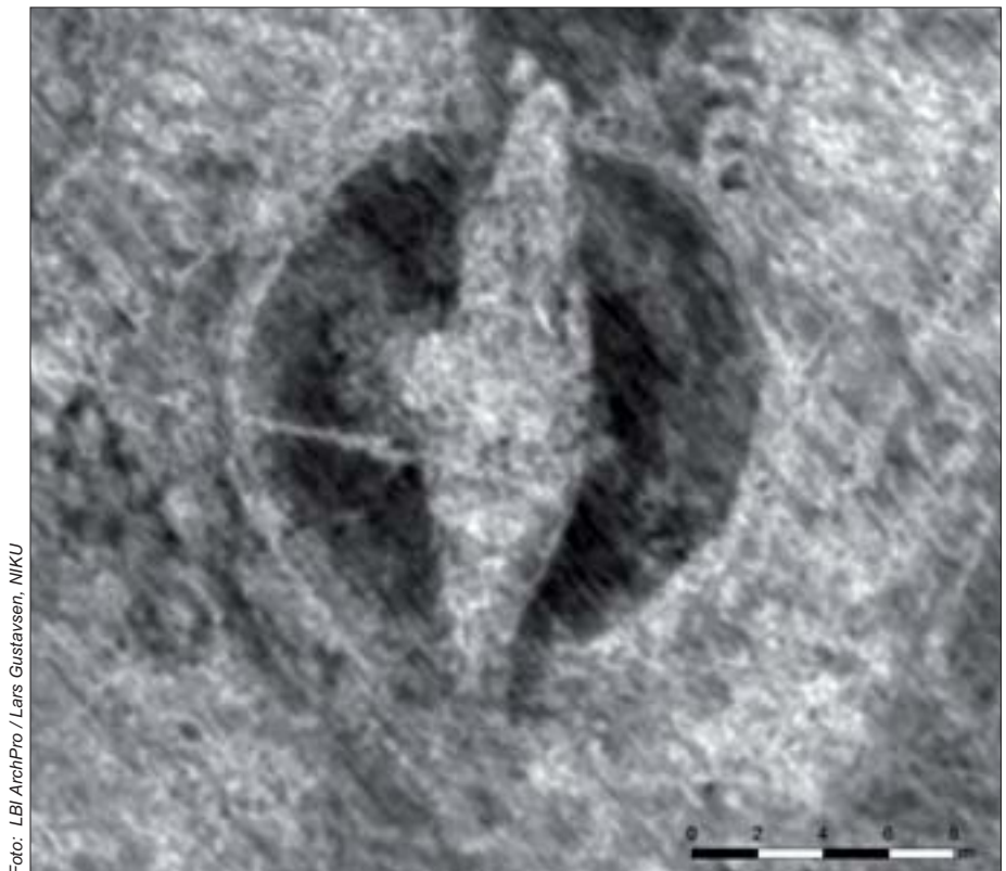
Die Umrisse des Wikingerschiffes sind in dieser Animation der Radardaten deutlich zu sehen.
