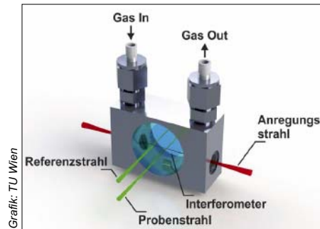
Eine schematische Darstellung der Meßzelle, entwickelt an der TU Wien
