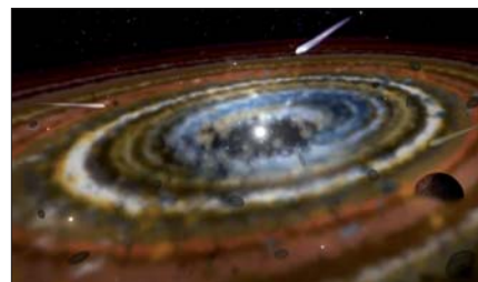
Drei Exoplaneten entdeckt
