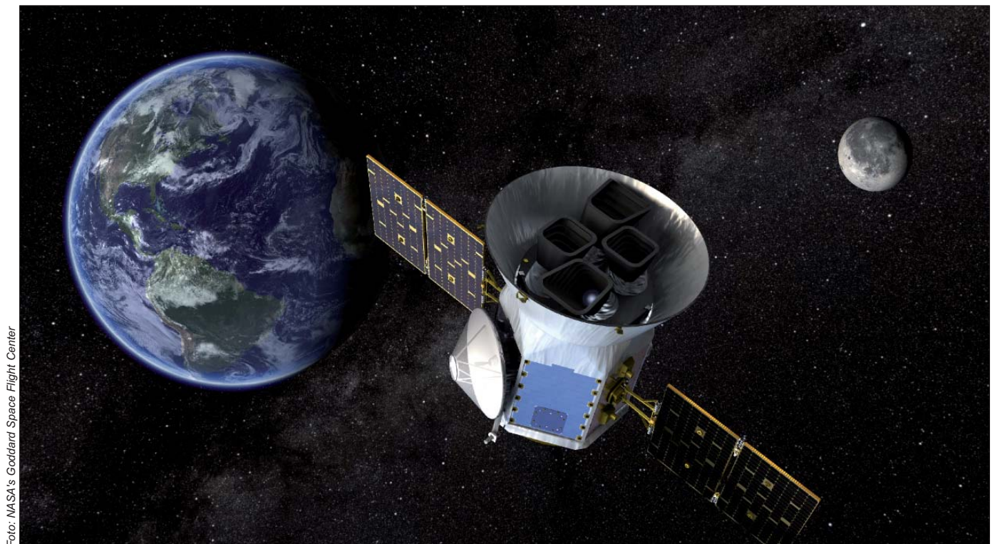
Das Weltraumteleskop der NASA, TESS (Transiting Exoplanet Survey Satellite), ist seit April 2018 auf der Suche nach Exoplaneten – und hat nun Exokometen entdeckt (Illustration).
