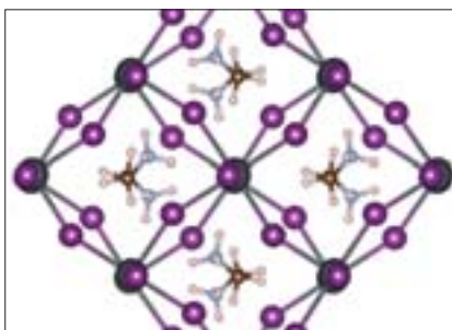
Hochsymmetrische Atomstruktur von MAPbI 3 bei Raumtemperatur.
