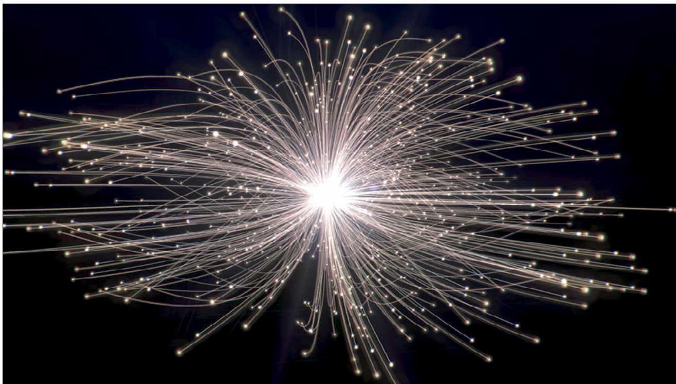
Künstlerischer Blick auf ein Kollisionsereignis bei der FCC
