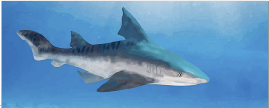
Rekonstruktion des Trias Meeresfisches Acrodon
